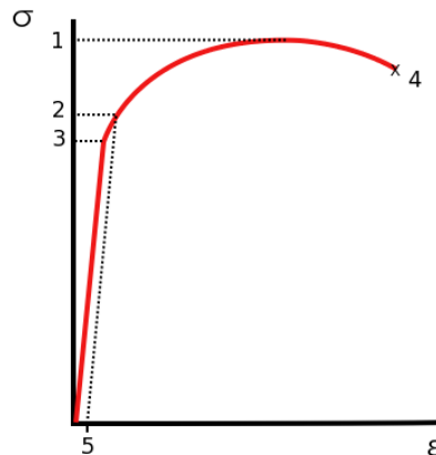
Figura 2.- Curva de tensión frente a deformación típica del aluminio. 1.-Resistencia a la tracción máxima. 2.-Resistencia al rendimiento (Yield Point). 3.-Tensión límite proporcional. 4.-Fractura. 5.-Tensión de compensación (típicamente 0.2%).
