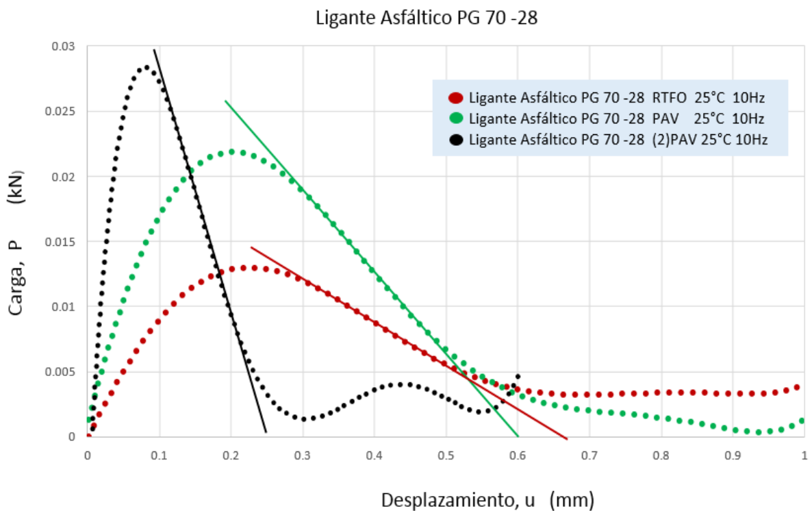
Figura 14.- Gráfica Carga-Desplazamiento del ligante asfáltico PG 70-28 después de RTFO, después de PAV y después de dos veces PAV utilizando el método propuestos en este estudio.
