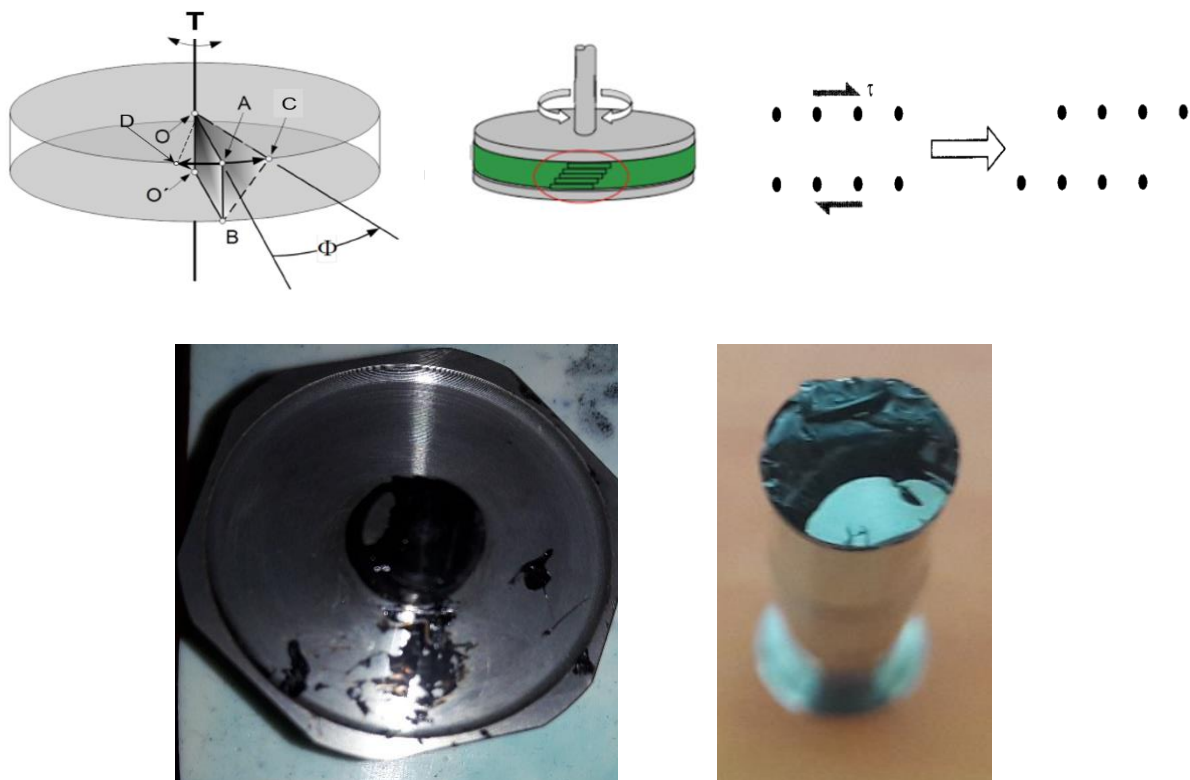
Figura 7.- Comprobación de la determinación del área de fractura ( \text{área} = 0.5 \cdot \text{radio}^2 \cdot \Phi ) para determinación del de la energía de fractura utilizando este método de prueba.
