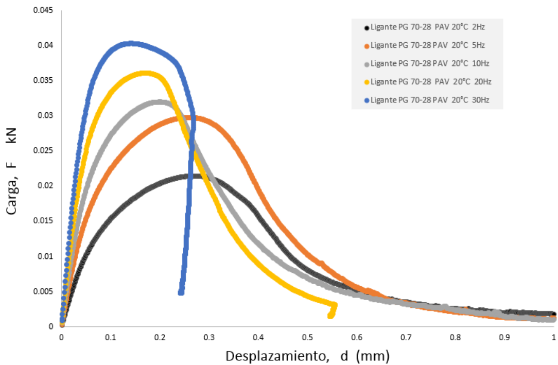
Figura 27.- Curva Carga-desplazamiento del ligante asfáltico PG 70-28 después de PAV a 20°C pero con diferentes frecuencias.
