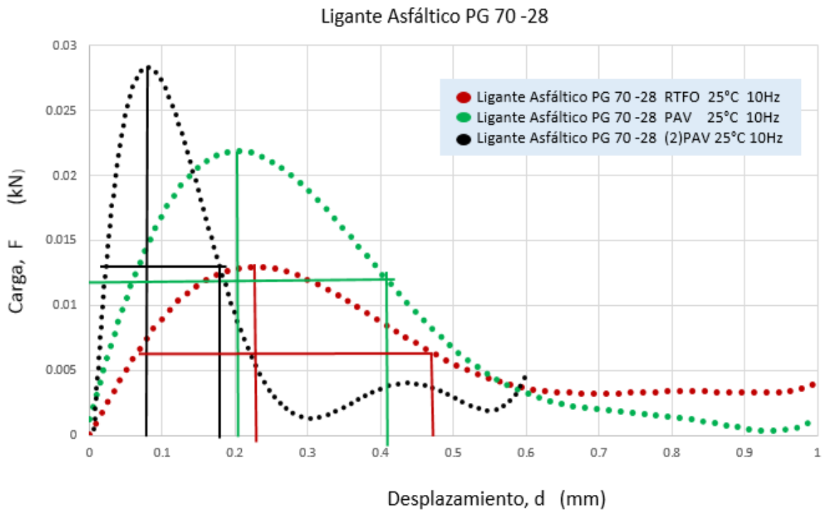
Figura 21.- Gráfica Carga-Desplazamiento del ligante asfáltico PG 70-28 después de RTFO, después de PAV y después de dos veces PAV utilizando el método propuestos en este estudio y el procedimiento FENIX.
