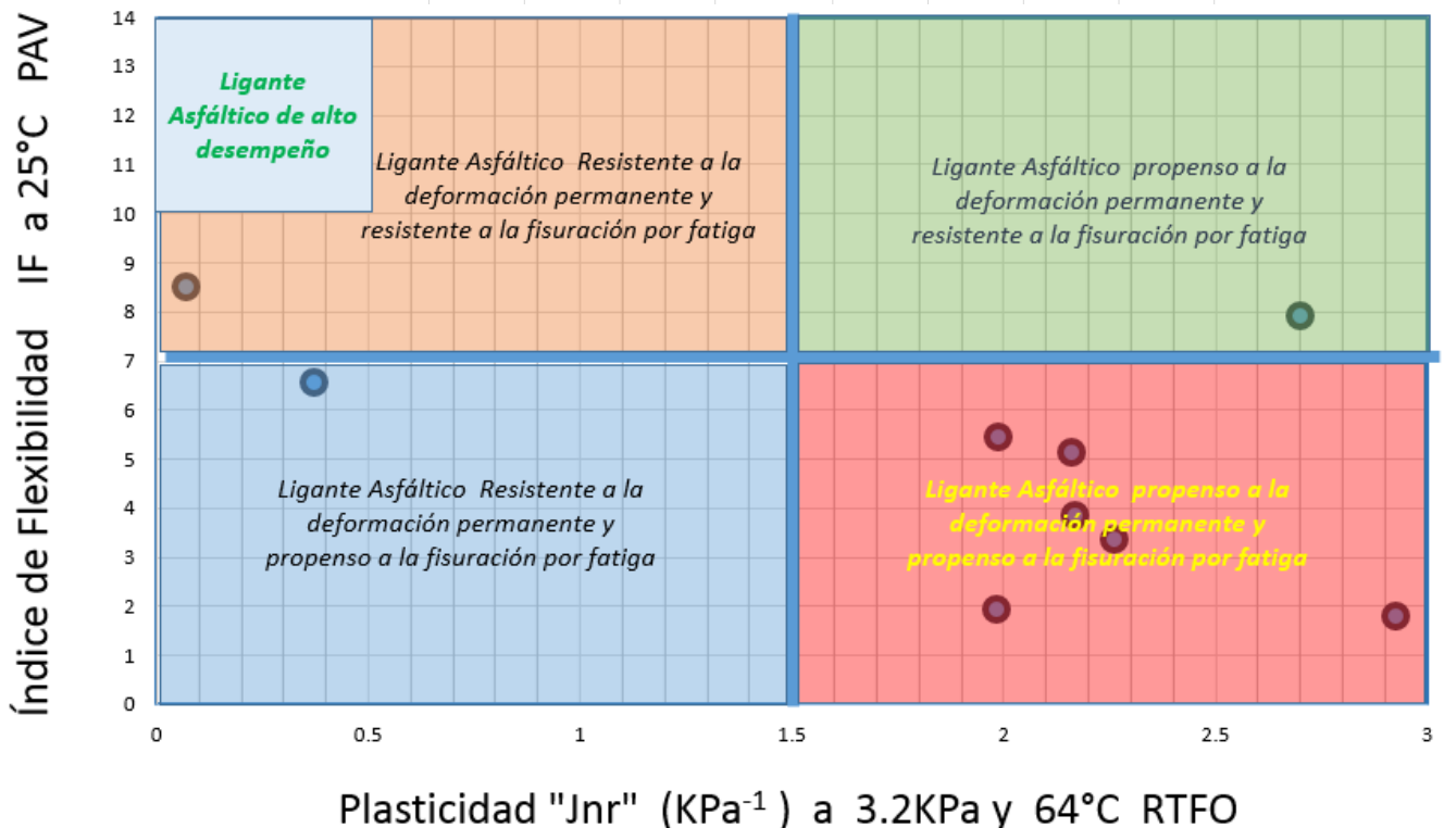
Figura 31.- Gráfica para la selección de un ligante asfáltico resistente a la fisuración por fatiga (alto Índice de Flexibilidad) y resistente a la deformación permanente (bajo valor de Plasticidad Jnr a 3.2KPa).
