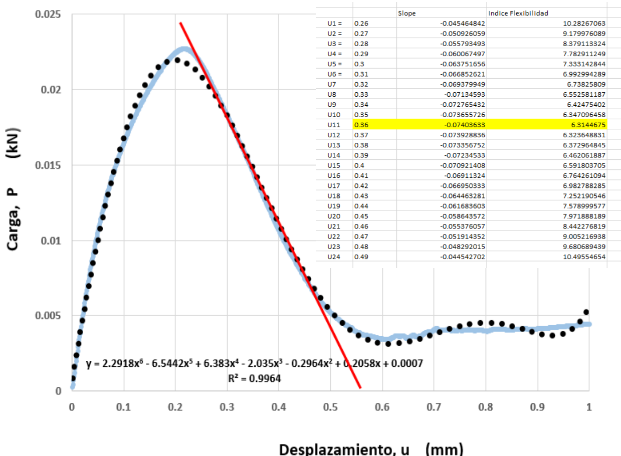
Figura 10.- Gráfica Carga-Desplazamiento del ligante asfáltico grado PG 76-22 después de RTFO
