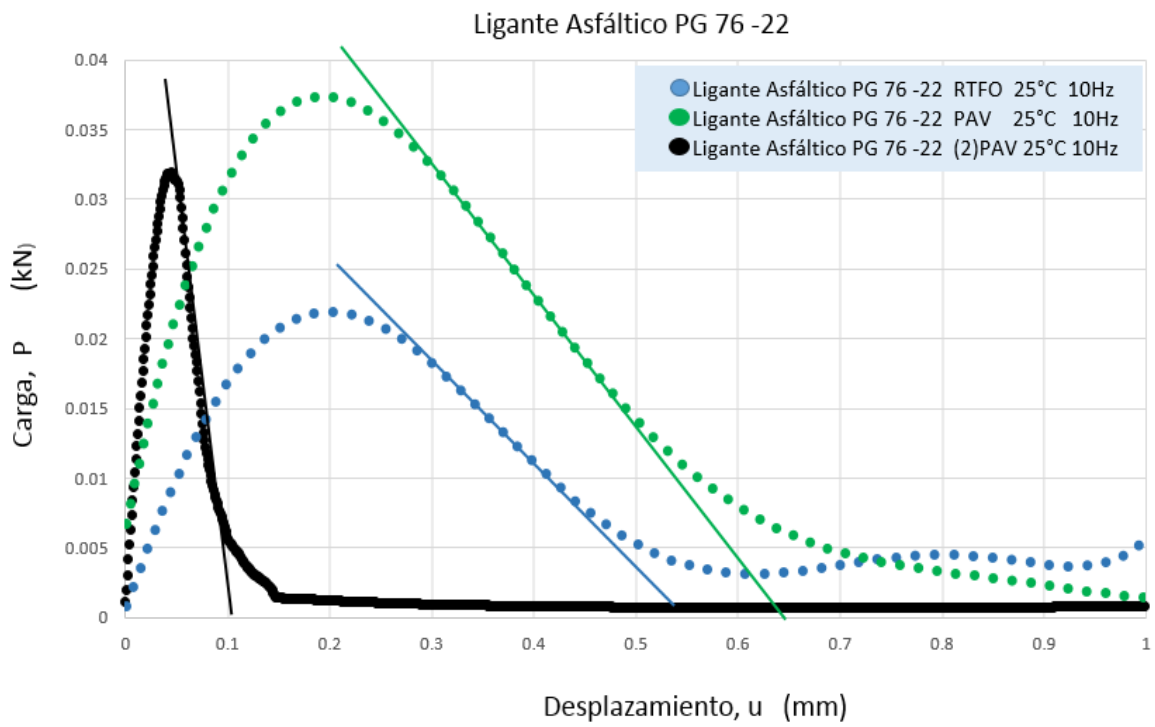
Figura 13.- Gráfica Carga-Desplazamiento del ligante asfáltico PG 76-22 después de RTFO, después de PAV y después de dos veces PAV utilizando el método propuestos en este estudio.
