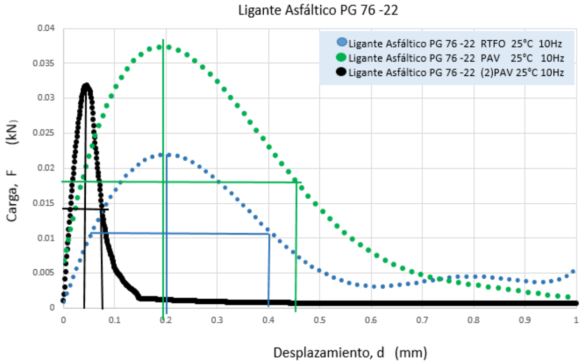
Figura 20.- Gráfica Carga-Desplazamiento del ligante asfáltico PG 76-22 después de RTFO, después de PAV y después de dos veces PAV utilizando el método propuestos en este estudio y el procedimiento FENIX.
