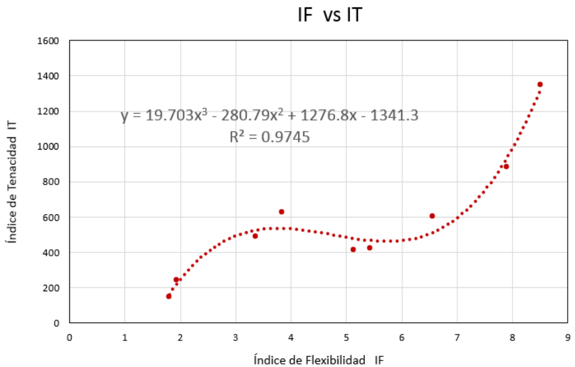
Figura 24.- Comparación polinomial entre el Índice de Flexibilidad y el Índice de Tenacidad de diferentes asfaltos después de PAV.
