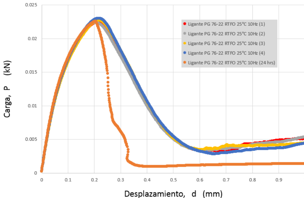
Figura 30.- Curva Carga-desplazamiento del ligante asfáltico PG 76-22 después de RTFO por cuadruplicado con un tiempo de reposo de 2 horas como máximo y una muestra de este ligante con un tiempo de reposo de 24 horas.
