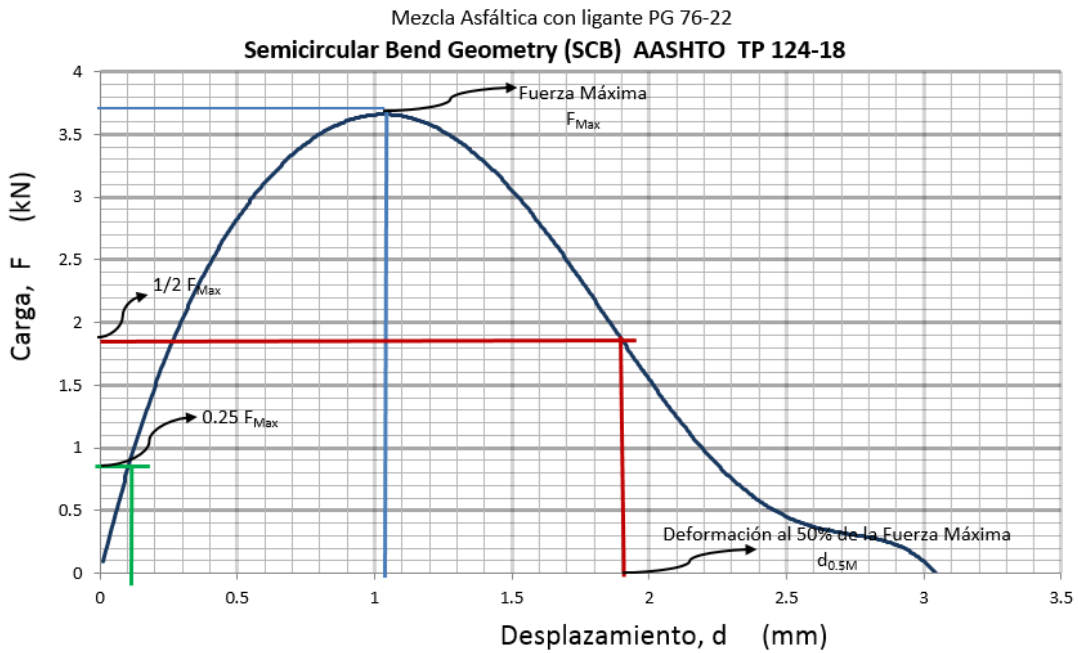
Figura 17.- Gráfica Carga-Desplazamiento de la mezcla asfáltica fabricada con el ligante asfáltico PG 76-22 utilizando el método AASHTO TP 124-18 (Semi-Circular Bending Test "SCB") y mostrando los parámetros del procedimiento Fenix.
