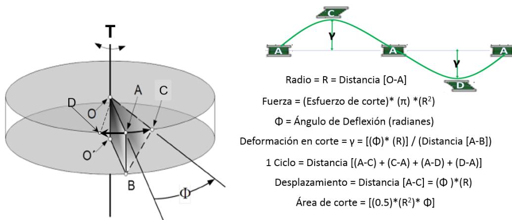
Figura 4.- Movimiento del plato superior durante la prueba del método propuesto.
