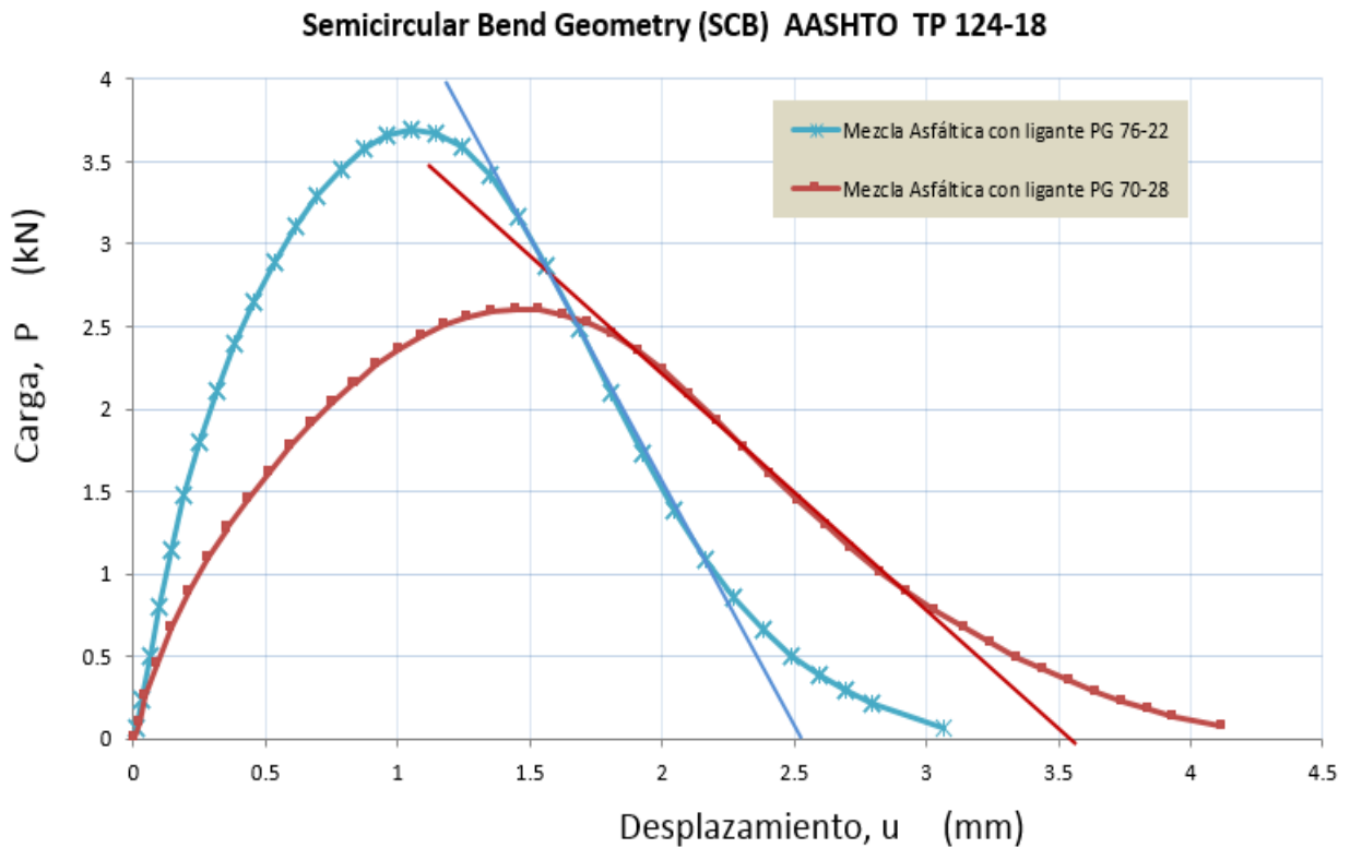
Figura 12.- Gráfica Carga-Desplazamiento de las mezclas asfálticas fabricadas con los ligantes asfálticos PG 76-22 y PG 70-28 utilizando el método AASHTO TP 124-18 (Semi-Circular Bending Test "SCB").
