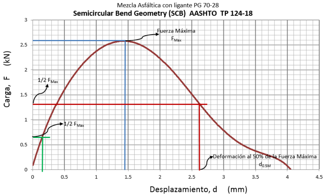
Figura 19.- Gráfica Carga-Desplazamiento de la mezcla asfáltica fabricada con el ligante asfáltico PG 70-28 utilizando el método AASHTO TP 124-18 (Semi-Circular Bending Test "SCB") y mostrando los parámetros del procedimiento Fenix
