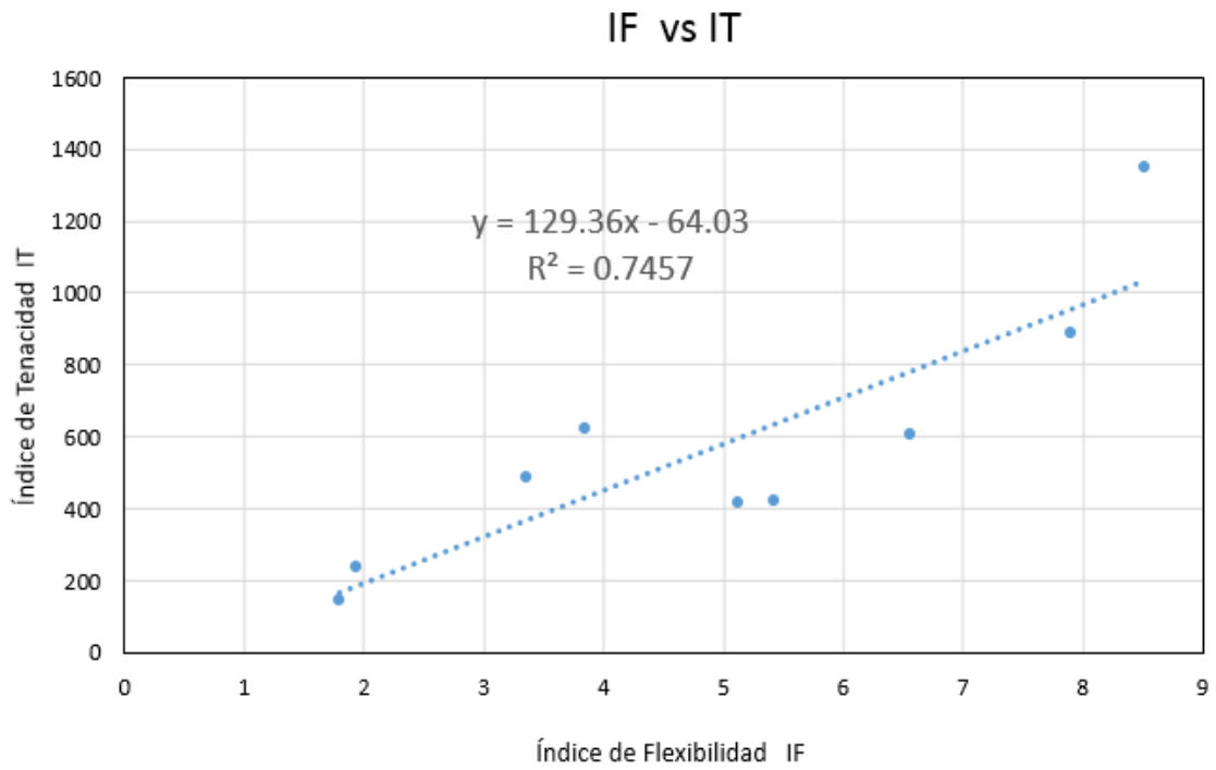
Figura 23.- Comparación lineal entre el Índice de Flexibilidad y el Índice de Tenacidad de diferentes asfaltos después de PAV.
