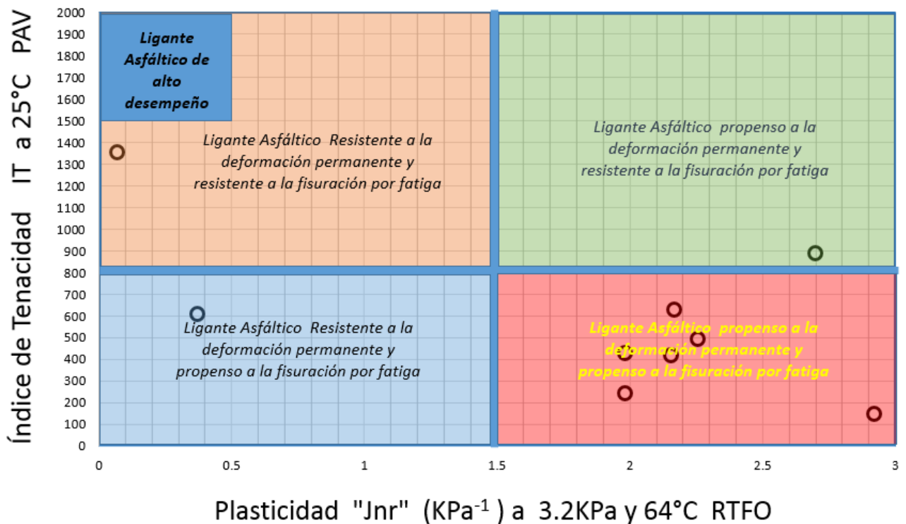
Figura 32.- Gráfica para la selección de un ligante asfáltico resistente a la fisuración por fatiga (alto Índice de Tenacidad) y resistente a la deformación permanente (bajo valor de Plasticidad "Jnr" a 3.2KPa).
