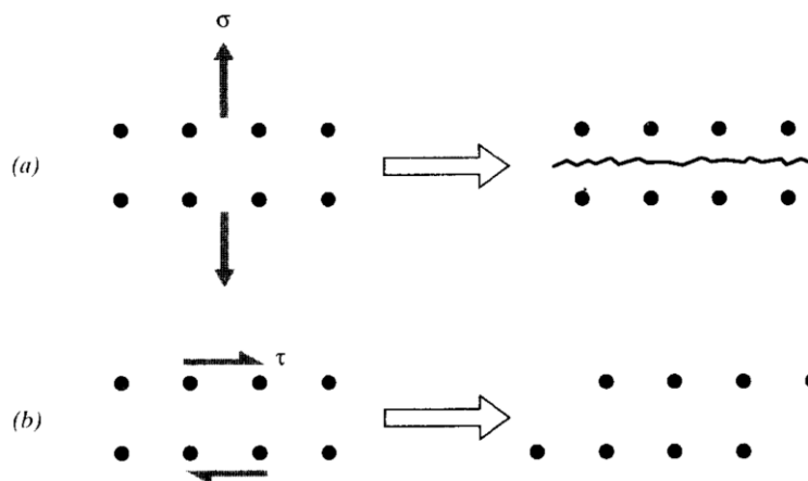
Figura 6.- La fractura es causada por un esfuerzo de tensión (a) y el deslizamiento es causado por un esfuerzo cortante (b) por lo que ambos esfuerzos pueden conducir a la fractura.
